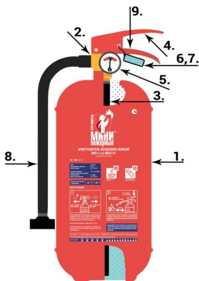
Рисунок 1. Общий вид конструкции огнетушителя
